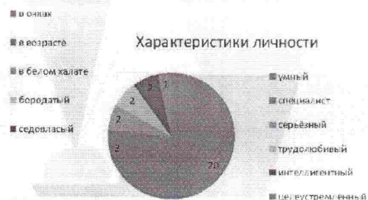
К. Циолковский 2/1
